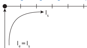
Einspeisung am Schienenanfang bzw. -ende Feeding at beginning or end of bar
