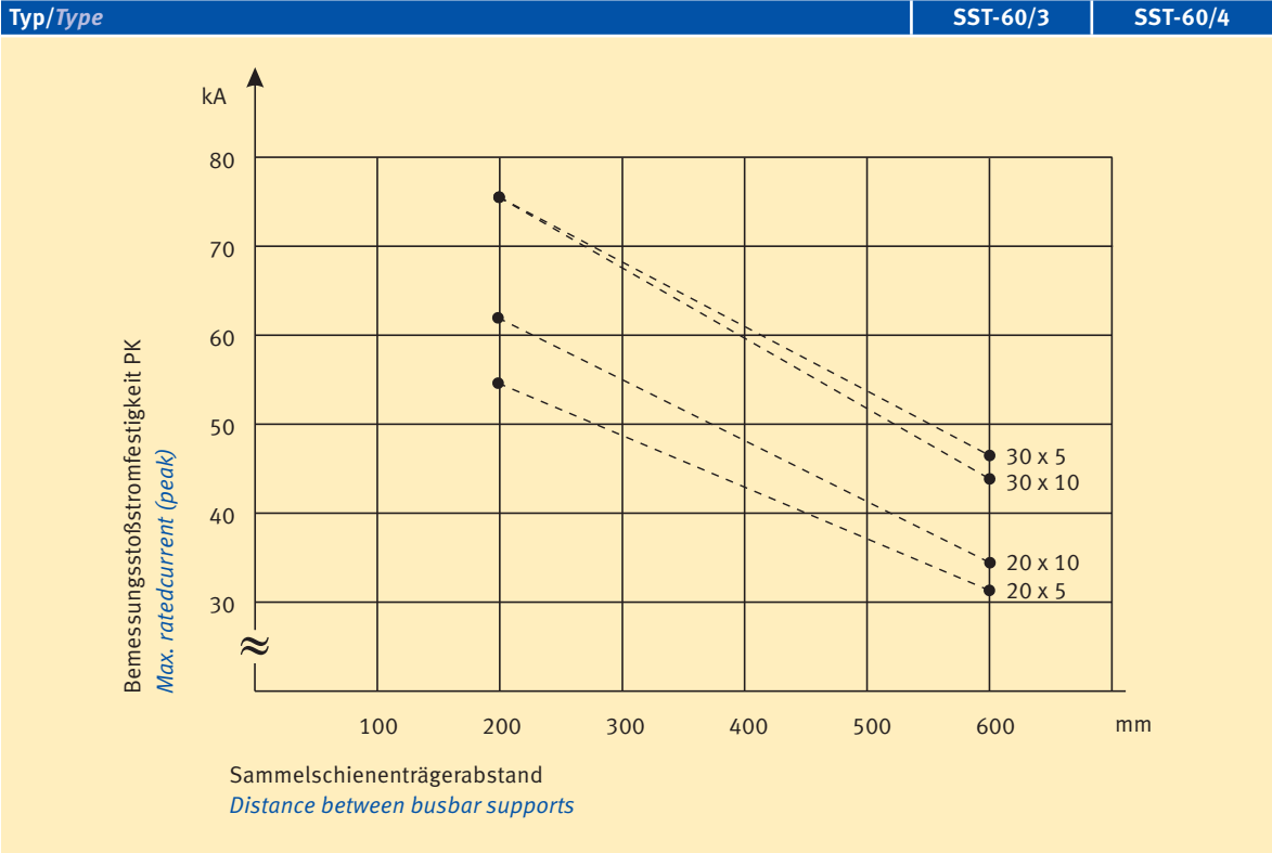
Bemessungsstoßstromfestigkeit I_{PK} des Sammelschienträgers in Abhängigkeit vom Sammelschienträgerabstand Max. rated current I_{PK} of the busbar support depending on the busbar support spacing
